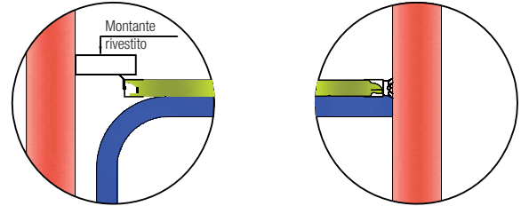
Montaggio in luce
