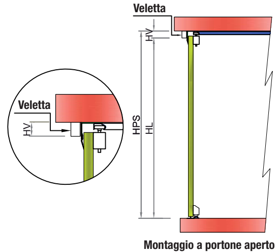
Montaggio in luce
