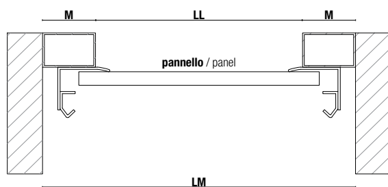
SEZIONE ORIZZONTALE MONTAGGIO IN LUCE HORIZONTAL SECTION LIGHT MOUNTING
