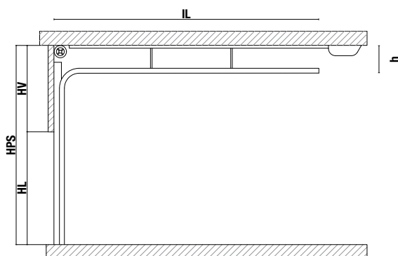
SEZIONE VERTICALE MONTAGGIO IN LUCE SEZIONE VERTICALE MONTAGGIO IN LUCE
