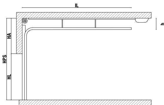
SEZIONE VERTICALE MONTAGGIO OLTRE LUCE SEZIONE VERTICALE MONTAGGIO OLTRE LUCE
