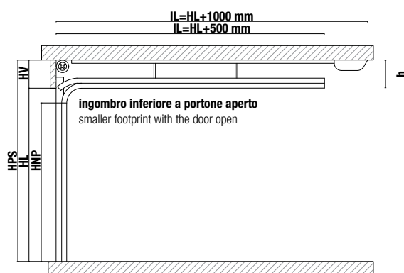
SEZIONE VERTICALE MONTAGGIO IN LUCE
