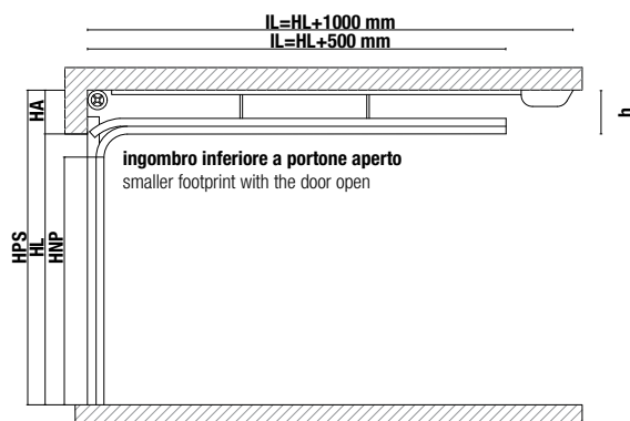
SEZIONE VERTICALE MONTAGGIO OLTRE LUCE VERTICAL SECTION ASSEMBLY BEYOND THE SPAN
