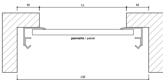
SEZIONE ORIZZONTALE MONTAGGIO OLTRE LUCE HORIZONTAL SECTION ASSEMBLY BEYOND THE SPAN
