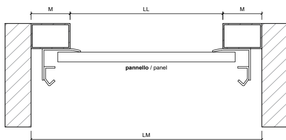
SEZIONE ORIZZONTALE MONTAGGIO IN LUCE HORIZONTAL SECTION ASSEMBLY LIGHT MOUNTING
