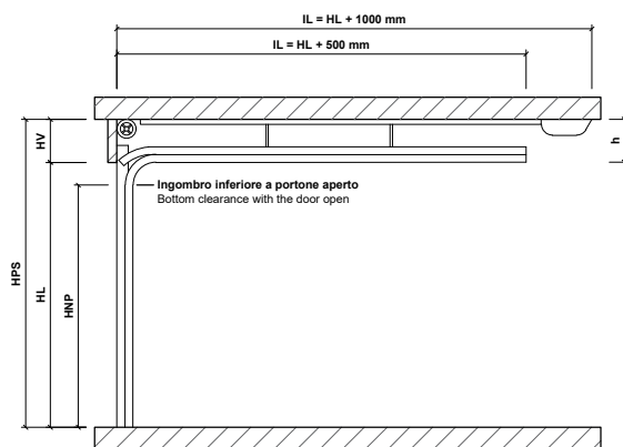
SEZIONE VERTICALE MONTAGGIO IN LUCE VERTICAL SECTION LIGHT MOUNTING
