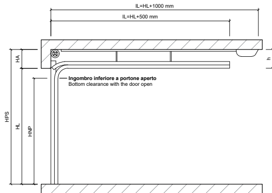
SEZIONE VERTICALE MONTAGGIO OLTRE LUCE VERTICAL SECTION ASSEMBLY BEYOND THE SPAN
